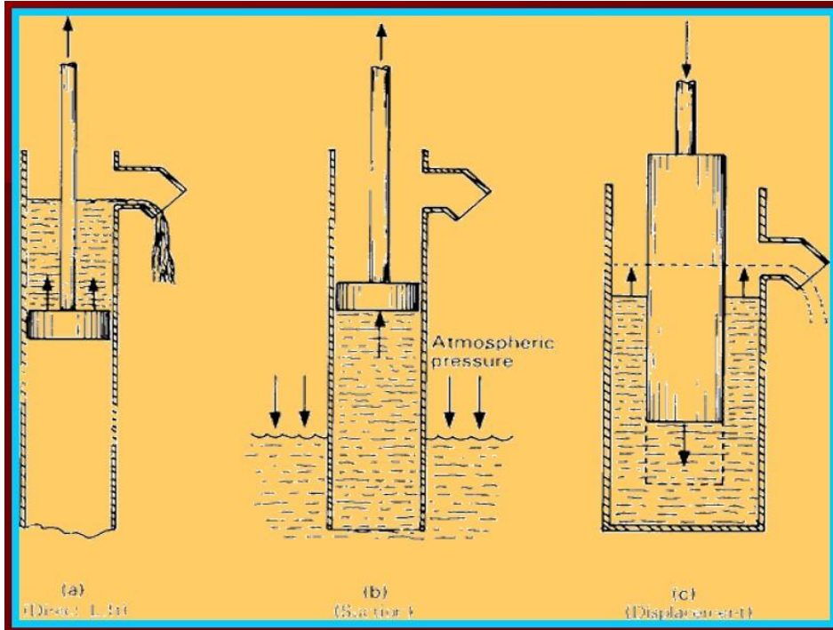
الشكل رقم (٥) - يبين الازاحة الإيجابية للمضخات
