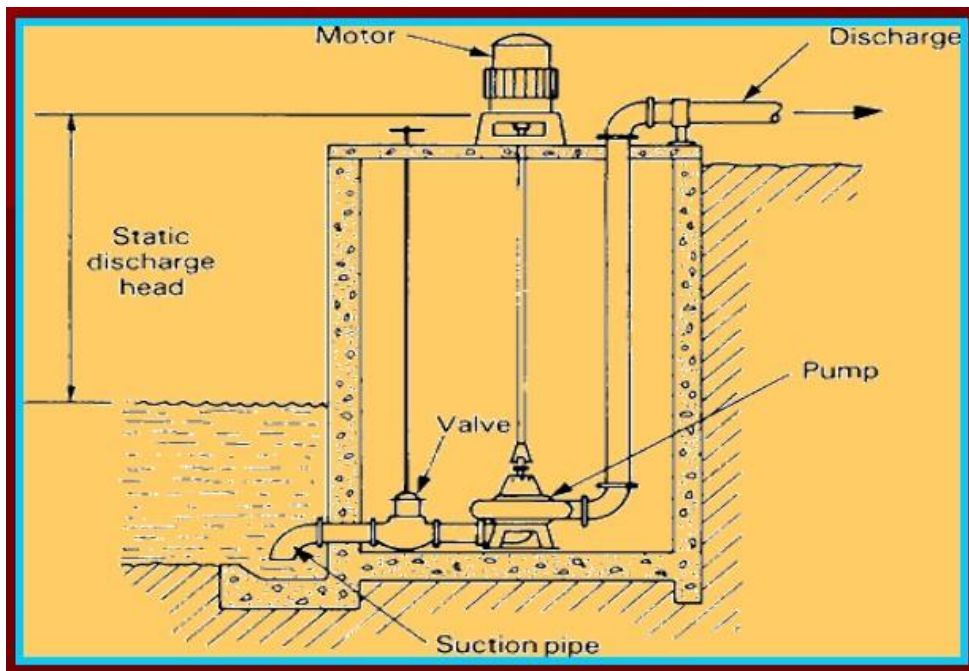
الشكل رقم (٦) - طريقة تثبيت مضخة الطرد المركزي تحت السطح
