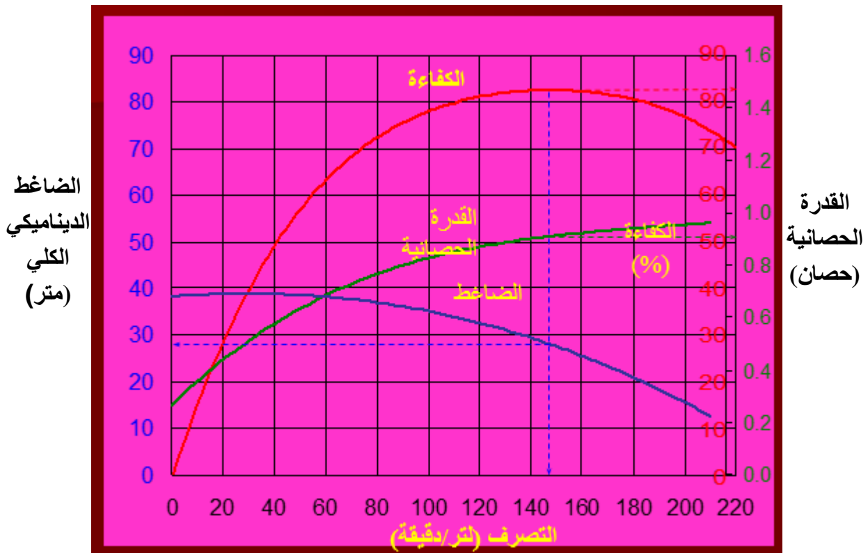
الشكل رقم (٧) - يبين جدول الأداء لمضخات الطرد المركزي
