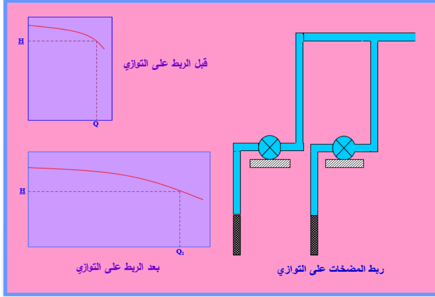
الشكل رقم (٩) - يبين أداء المضخات قبل وبعد الربط على التوازي
