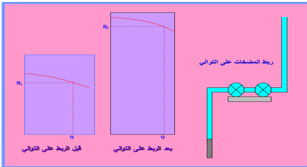
الشكل رقم (٨) - يبين أداء المضخات قبل وبعد الربط على التوالي
