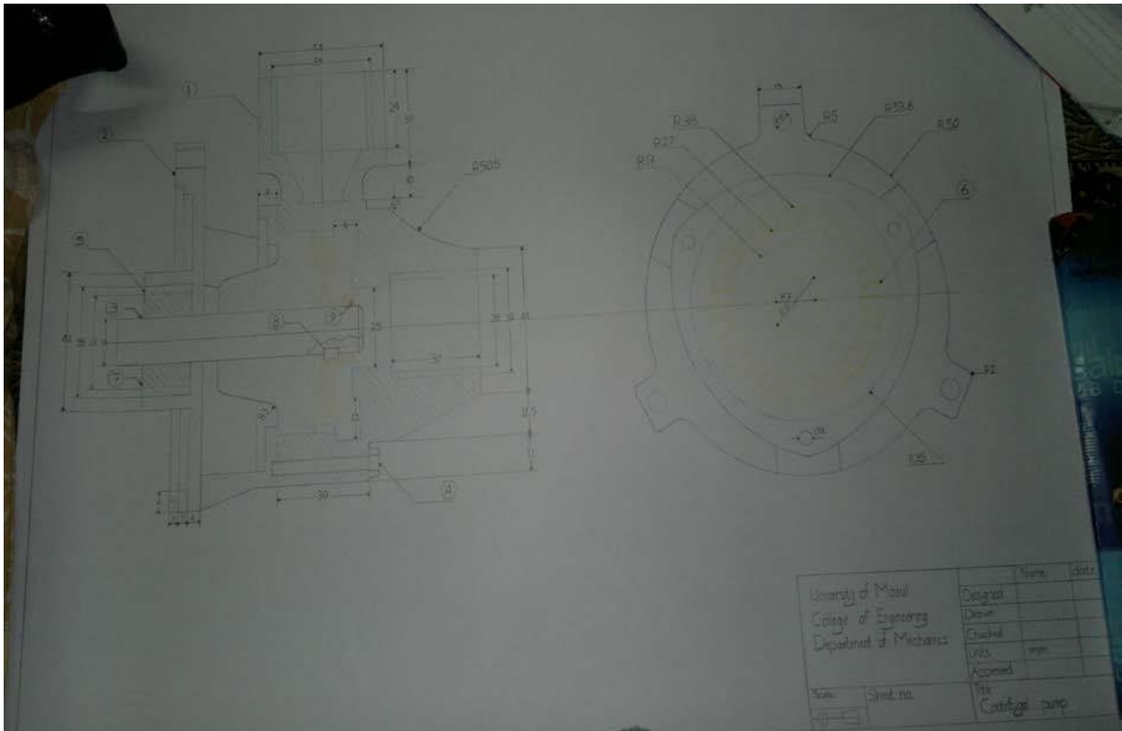
الشكل رقم (١٤) - يبين المقطعين العرضي والطولي للمضخة التي تم عملها
