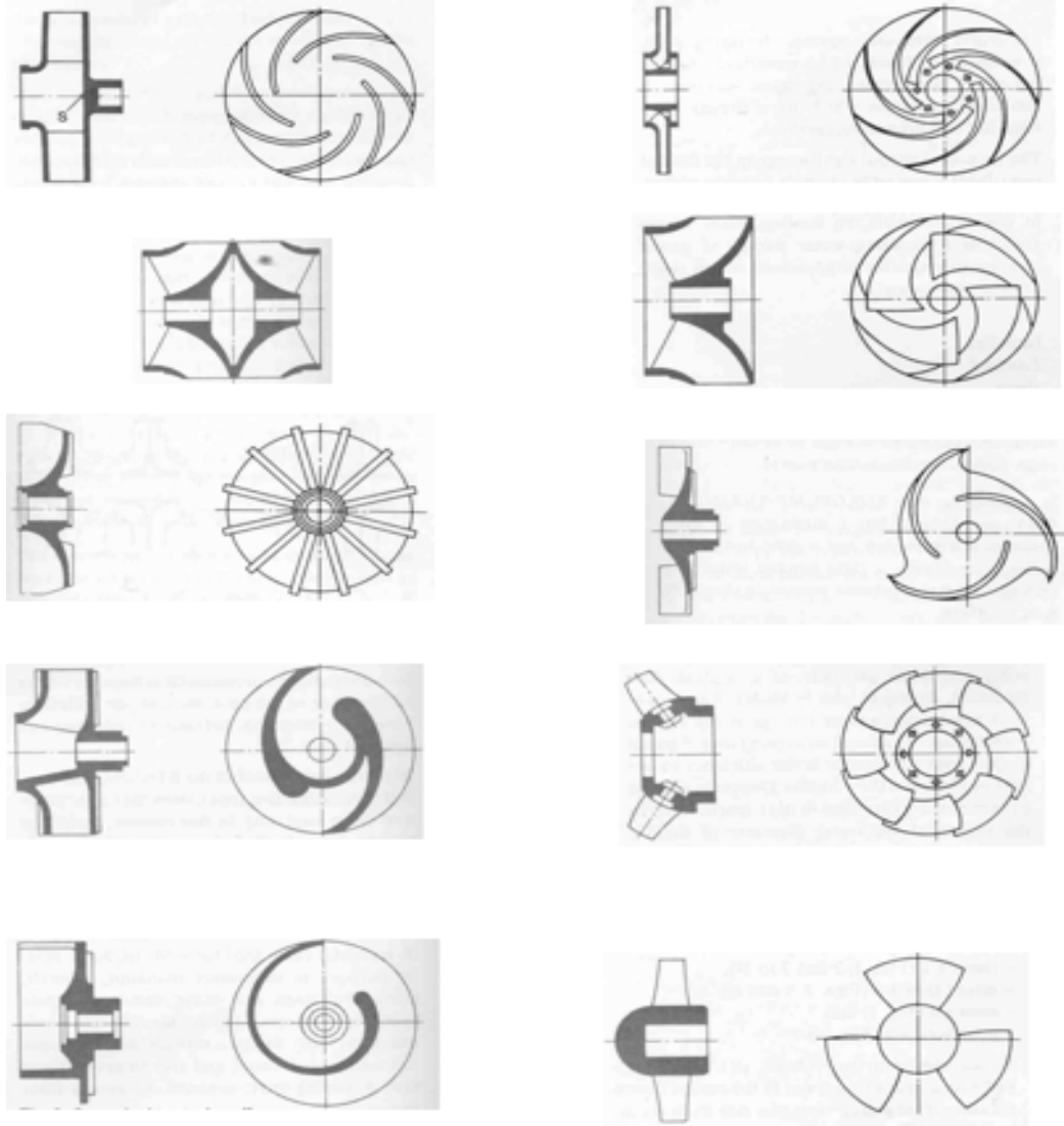
الشكل رقم (١١) - يبين أنواع مختلفة لشكل ريش مضخات الطرد المركزي
