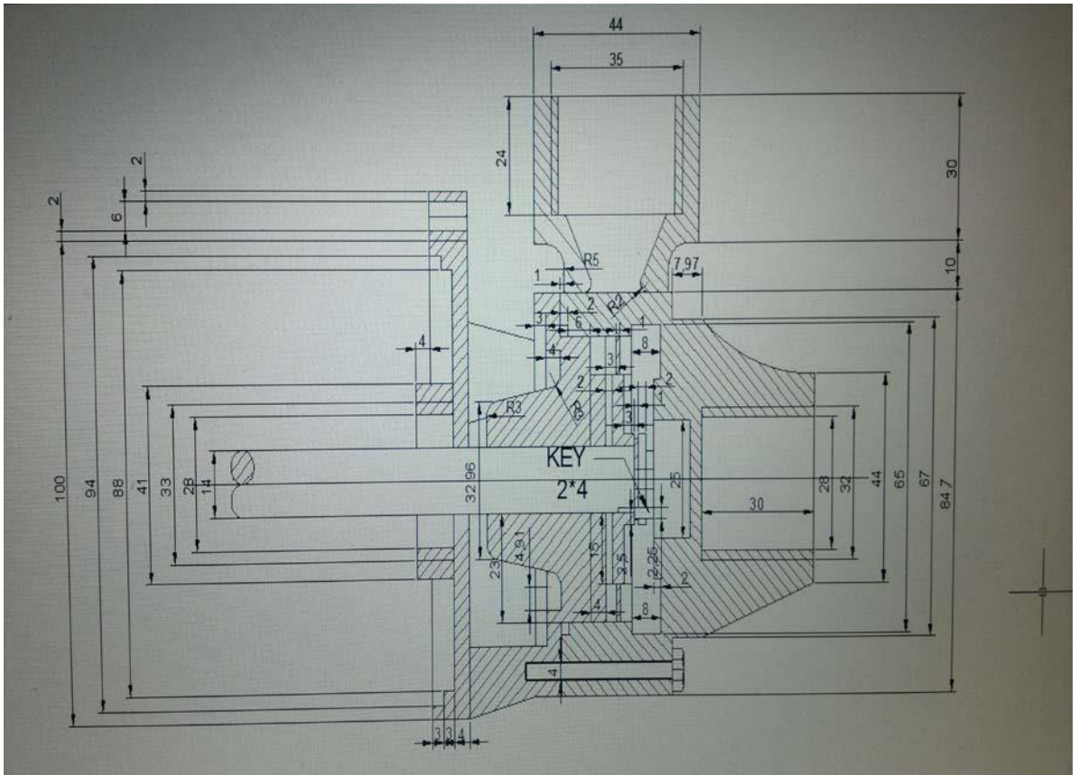
الشكل رقم (١٢) - يبين مقطع طولي لمضخة طرد المركزي التي تم عملها
